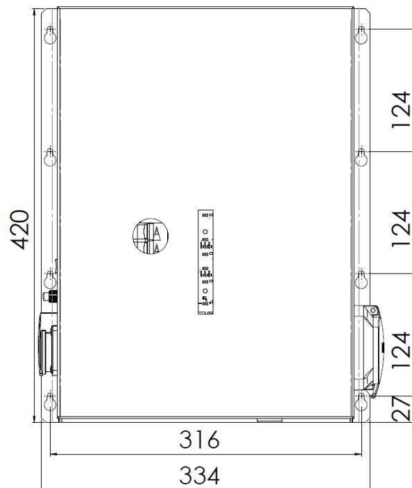
Kiinnitysreikien sijoittelu
