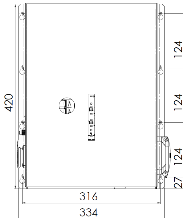
Fästhålens placering
